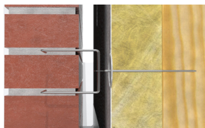
Montage av murkramla nr. 3 i murverkets liggfogar. Vertikalsnitt.
